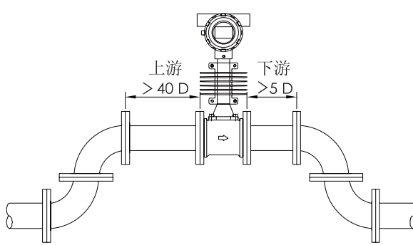
在同一个平面上有两个90°弯管
