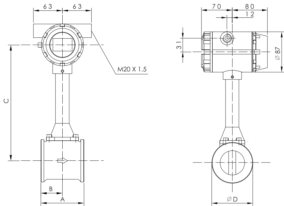
夹持型涡街流量计外形尺寸
