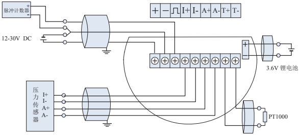
电池和 24V双供电 +使用脉冲输出 +压力传感器 +温度传感器
