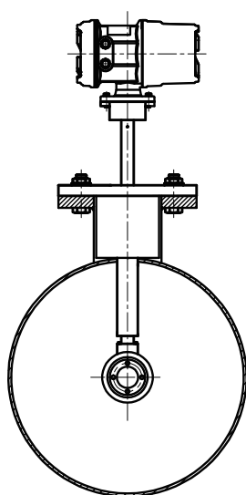
标准型法兰固定插入式电磁流量计
