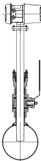
标准型在线插拔式电磁流量计
