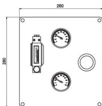
图 15 LZWB/1/M/RA/8/P
