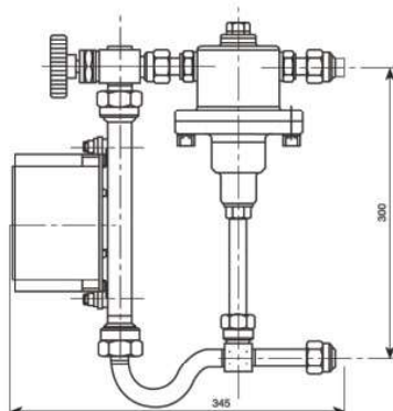
图 12 LZZ-( ) /D/RA/10/P
