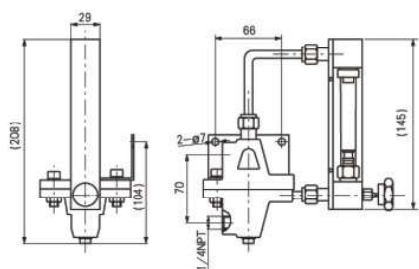
图 7 LZB-( ) DK/D/RE/8/P
