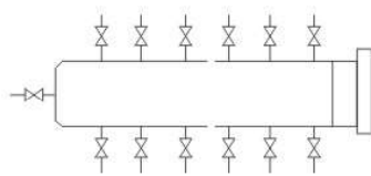
TKKFQ-II 型
