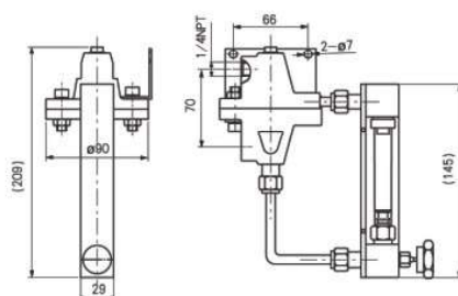
图 8 LZB-( ) DK/D/RA/8/P
