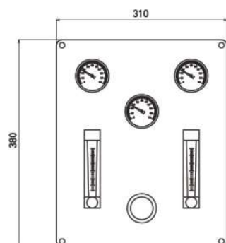
图 14 LZB-( ) DK/2/M/RA/8/P
