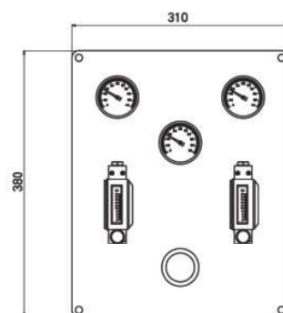
图 16 LZWB/2/M/RA/8/P
