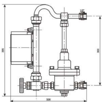
图 11 LZZ-( ) /D/RE/10/P
