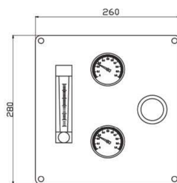
图 13 LZB-( ) DK/1/M/RA/8/P
