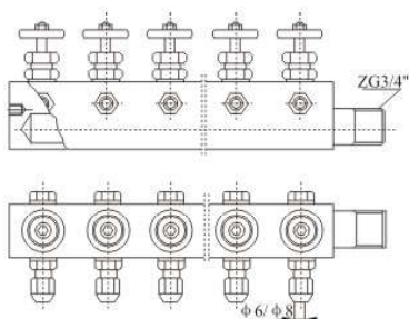
TKKFQ-III 型
