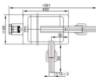
TKF1-24 沉降器(CJI 型气用) TKF1-24 Subside(use for gas)
