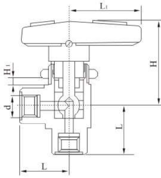
TKQ-5B Q13SA-64 型内螺纹角式球阀 TKQ-5B Q13SA-64 Female Angle Pattern Ball Valve
