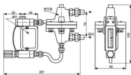
图 10 LZWB/D/RA/8/P
