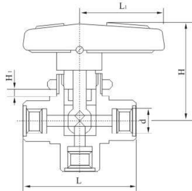
TKQ-6B Q14SA-64 型内螺纹三通球阀 TKQ-6B Q14SA-64 Femals Serew 3-Way Ball Valve
